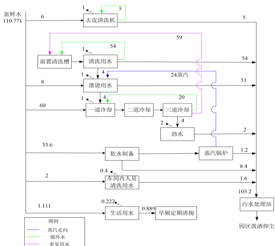
图 1 项目水量平衡图 单位: m 3 /d
