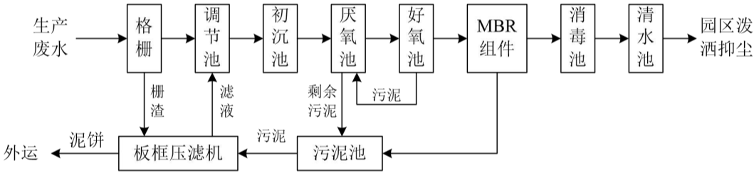
图4 污水处理站工艺流程及产排污节点图
