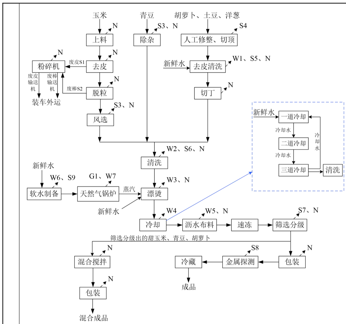
图 2 工艺流程及产排污节点图
