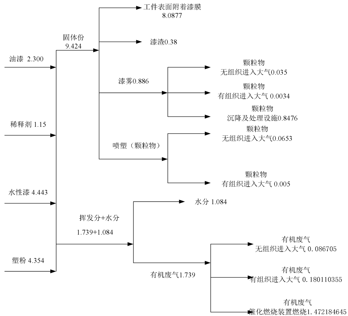
图1 漆料物料平衡图 单位 t/a
