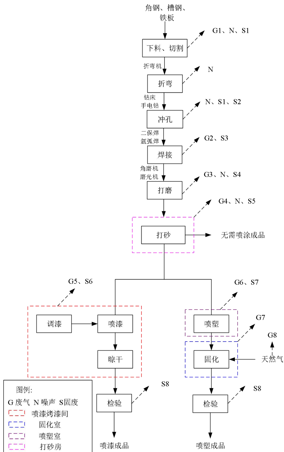
图 3 工艺流程及排污节点图
