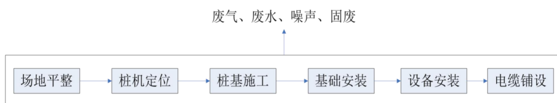
图 2-1 光伏阵列施工工艺及产污环节图
