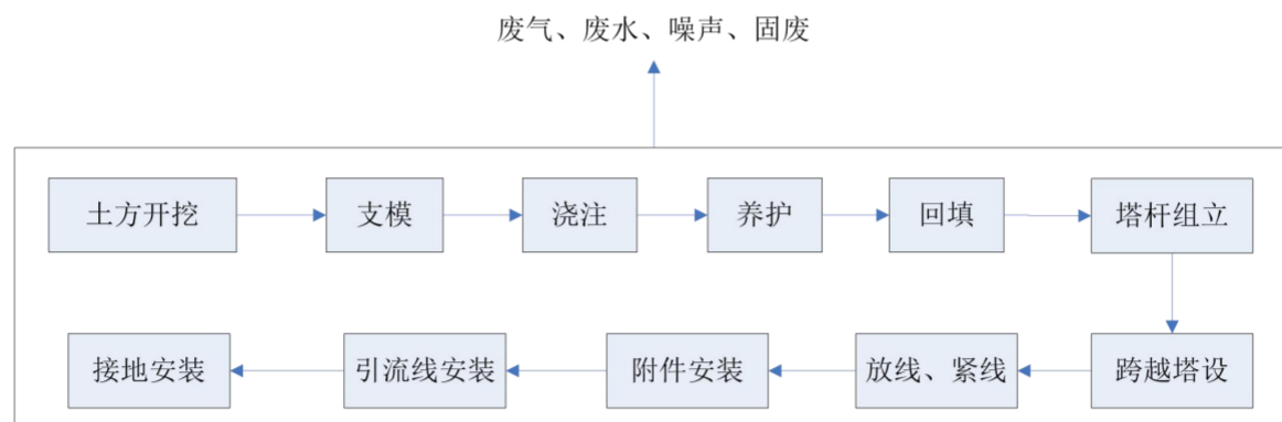
图 2-3 架空集电线路工艺及产污环节图
