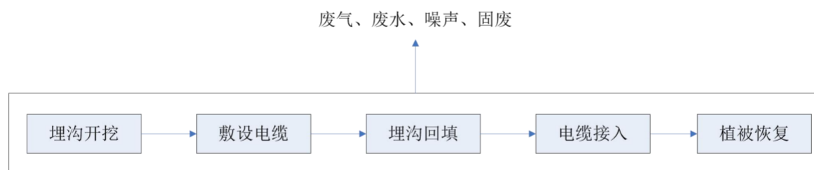
图 2-2 地埋集电线路工艺及产污环节图
