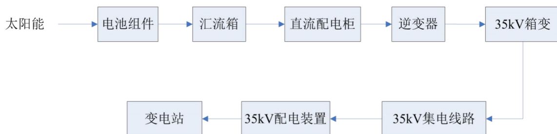
图2-5 运营期工艺流程图
