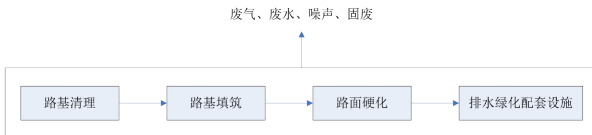
图 2-4 道路施工工艺流程图
