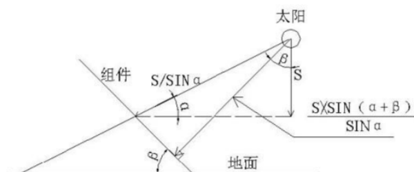
图 4-1 倾斜方阵面上的太阳总辐射量计算图
